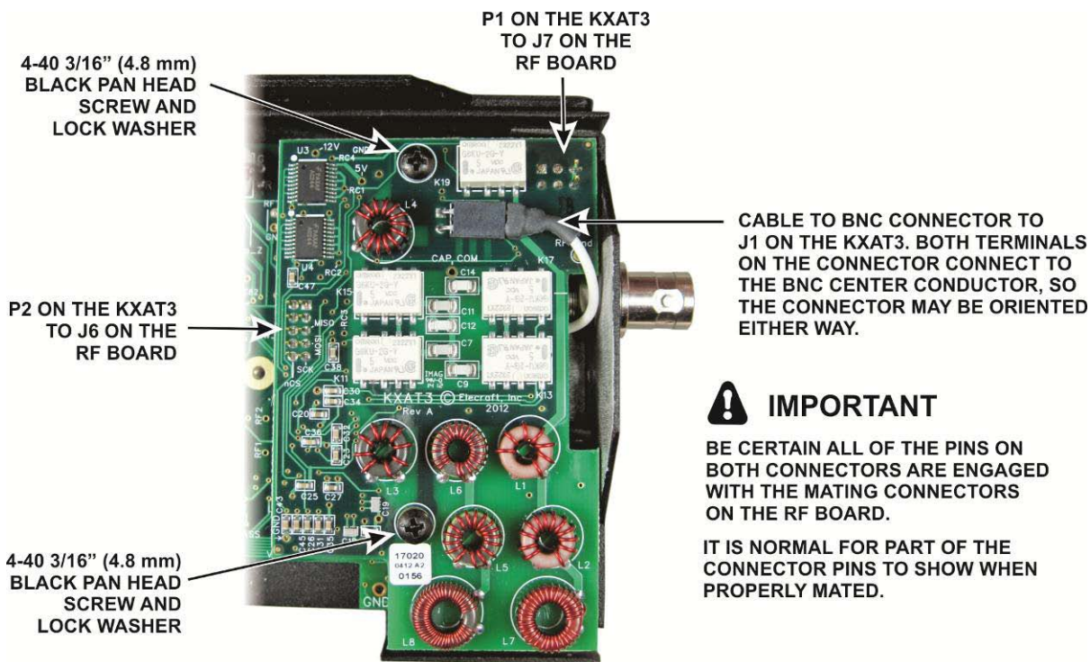
Figure 48. Installing the KXAT3 ATU.
